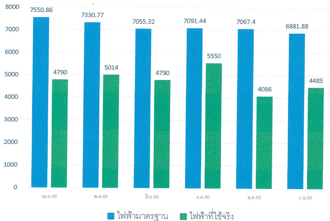
แผนภูมิแสดงการใช้ไฟฟ้าจริง เปรียบเทียบกับค่ามาตรฐานการใช้พลังงาน
